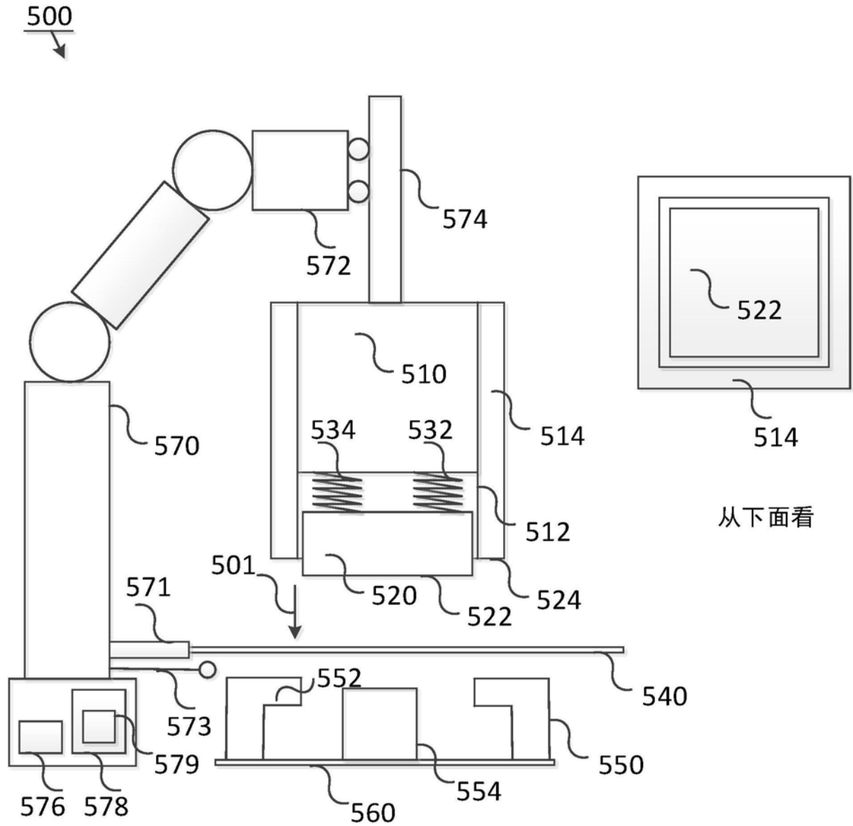
侧面图
